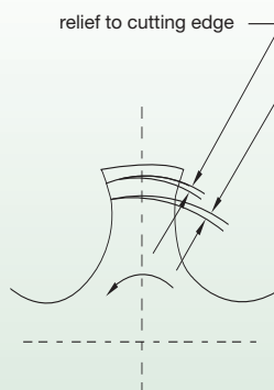
Eccentric Relief
