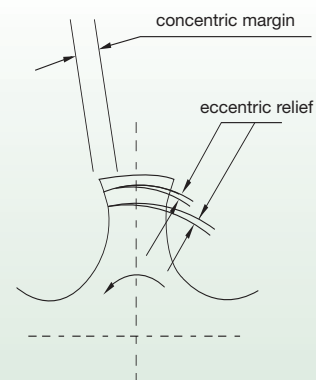
Con-Eccentric Relief
